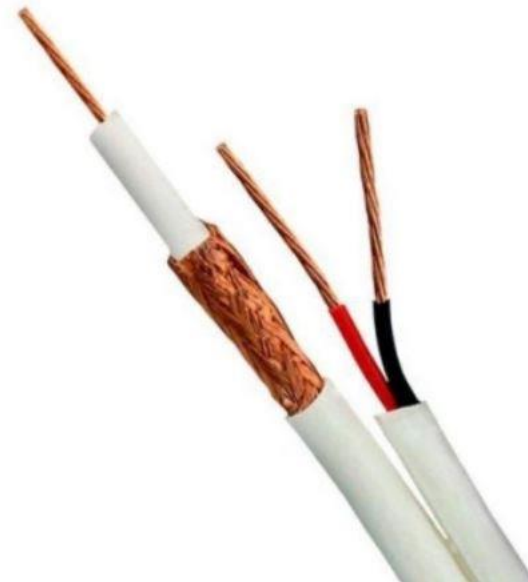
CABO COAXIAL BIPOLAR 80% DE MALHA Cód.: 4830052
