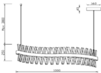
Cabo ajustável até 3000mm
