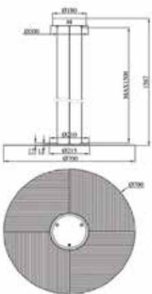
Cabo ajustável até 1500mm
