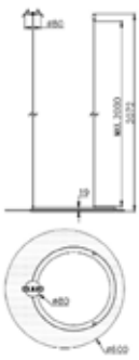
Cabo ajustável até 2000mm
