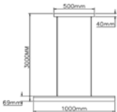
Cabo ajustável até 3000mm
