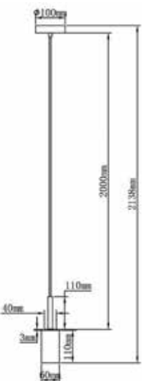
Cabo ajustável até 2000mm
