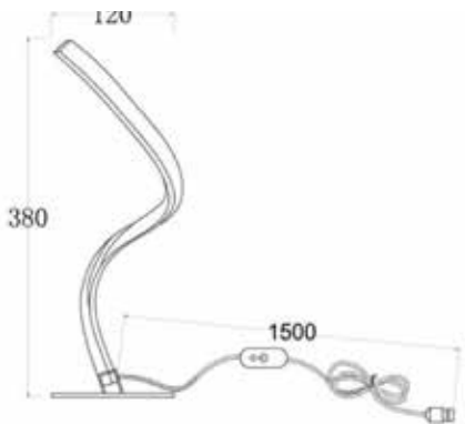
Cabo com 1500mm
