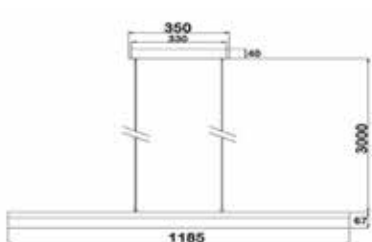
Cabo ajustável até 3000mm
