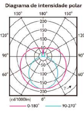
MC LEDtube IA 1200MM UO 16W865 T8
