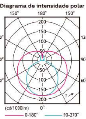
MC LEDtube IA 600mm HO 7W865 T8
