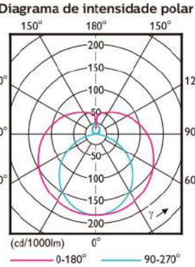
MC LEDtube IA 600mm HO 7W840 T8
