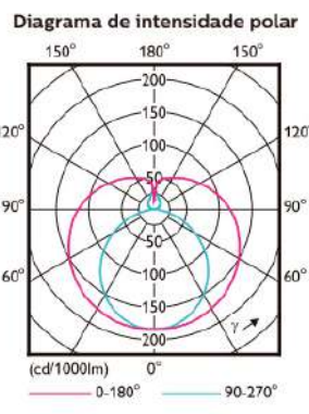
MC LEDtube IA 1200mm UO 16W840 T8
